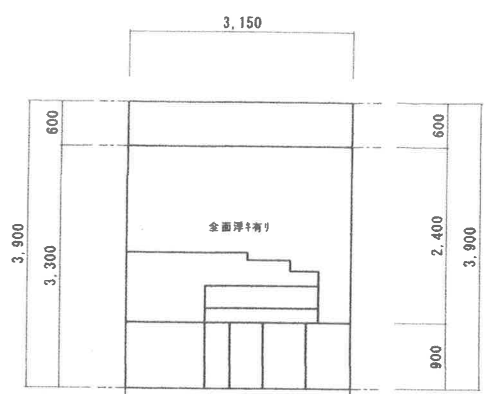
石蔵（小）南側B展開図
