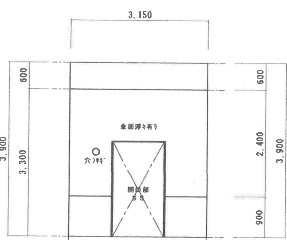
石蔵（小）北側D展開図
