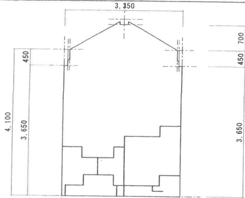
石蔵（大）西側A展開図
