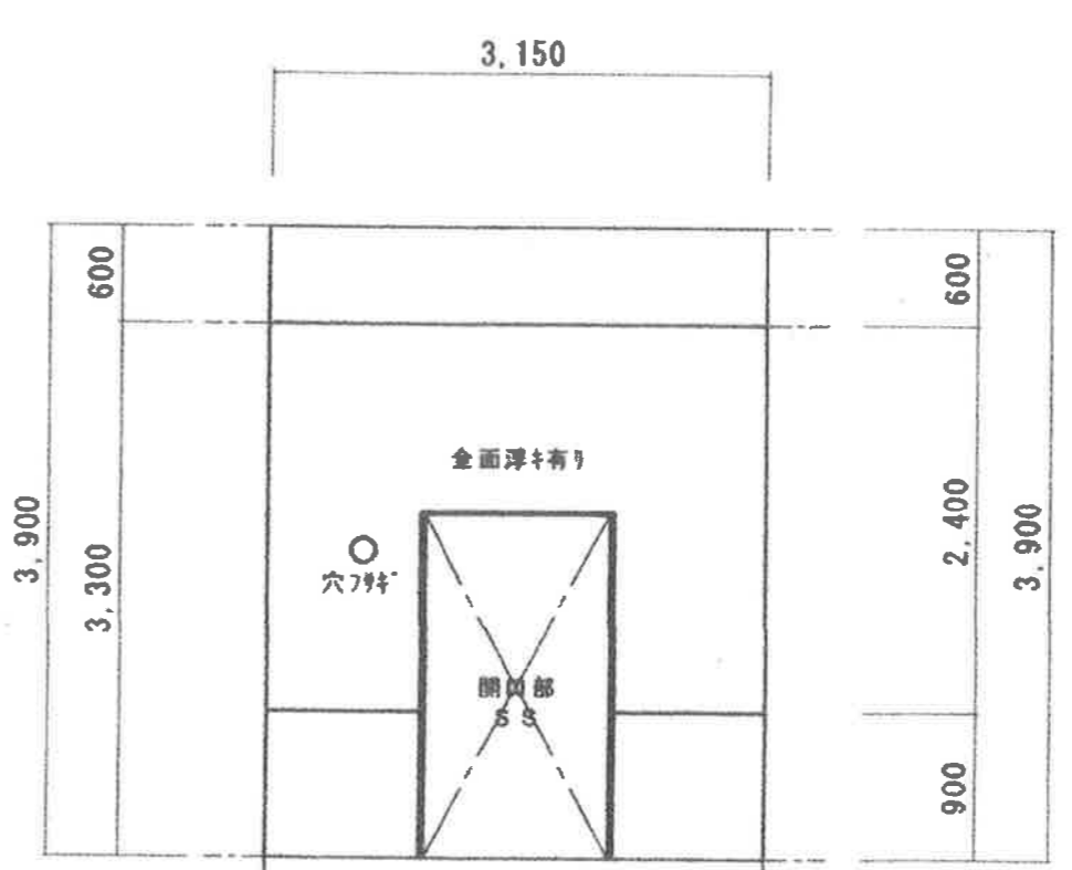
石蔵（小）北側D展開図
