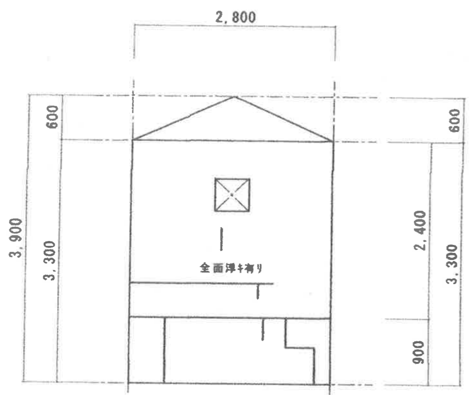
石蔵（小）西側A展開図
