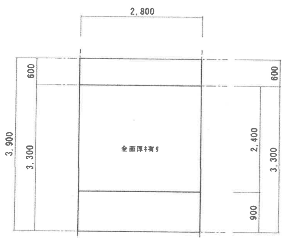
石蔵（小）東側C展開図
