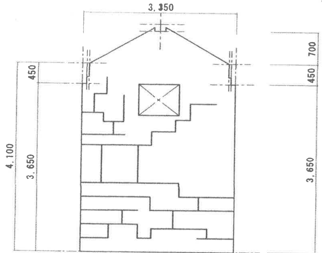
石蔵（大）西側A展開図
